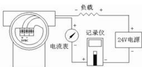
4~20mA 电流输出为二线制
