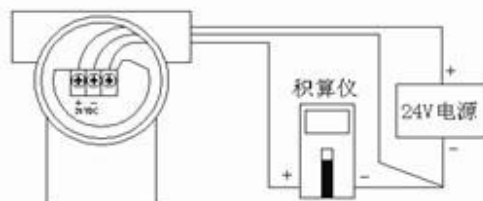
脉冲输出为二线制
